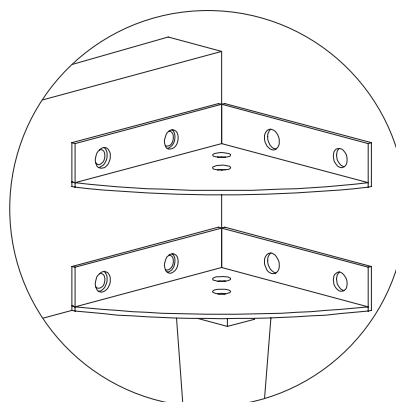
Dettaglio A, Scala 1:5 / Detail A, Scale 1:5
