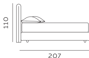
207 materasso lungh. cm. 190 mattress length cm. 190
